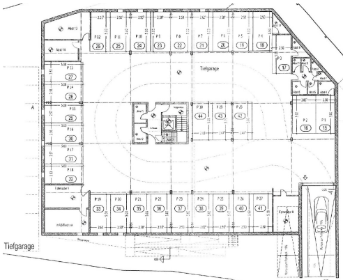
Grundriss Tiefgaragenstellplätze
