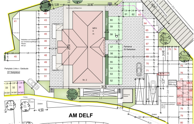
Grundriss Außenstellplätze
