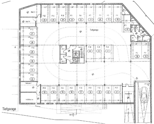
Grundriss Tiefgaragenstellplätze
